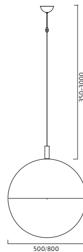
Vajerpendel/Wire pendant
