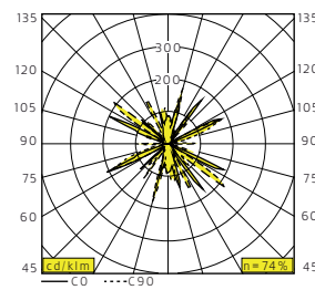
Pendelrör/Pendant tube
